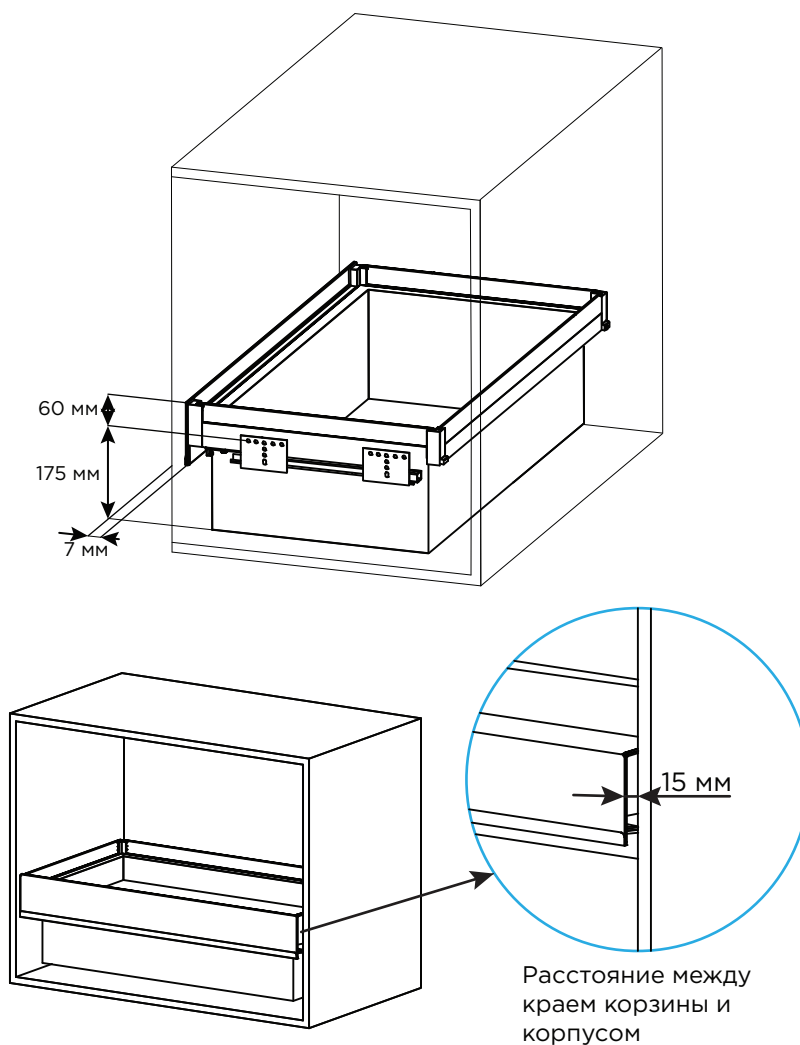
Схема системы, установленной в корпус
